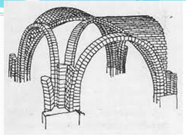
Ukázka vyzdívání žeber a pláště typické románské křížové klenby
